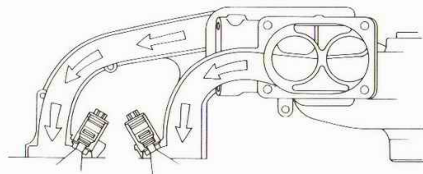
Computergesteuerte sequentielle elektronische Kraftstoffeinspritzung (SEFI).
