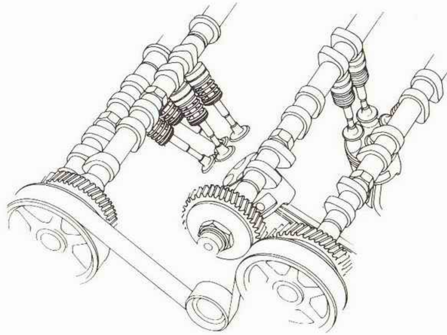
Optimaler Durchsatz mit vier Ventilen pro Zylinder.
