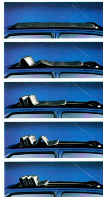
Das elektrische Faltschiebedach öffnet sich auf Knopfdruck.
